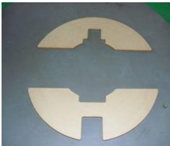
铁轭绝缘端圈
